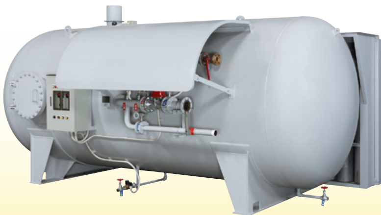
スプリンクラー消火設備用加圧送水装置（製品名「ナイアス」）
