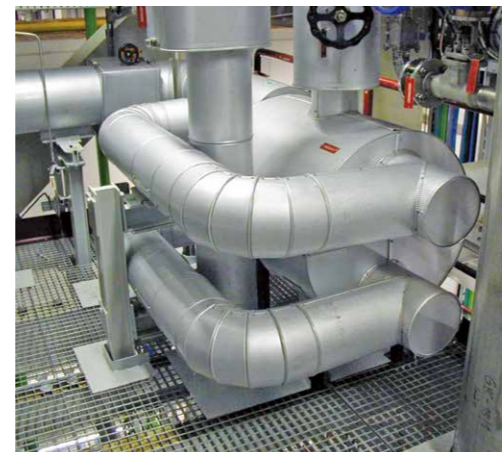
■温水加熱器 30MW (蒸気0.25MPa/DH-water 75/115℃)
