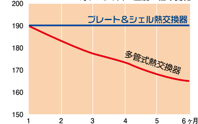
温度℃ 汚れによる出口温度の経年変化
